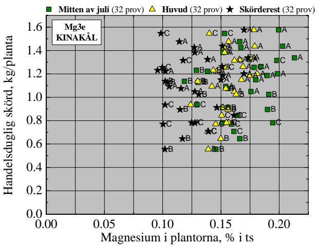
Figur Mg3a-g. Förhållandet mellan plantornas vikt och magnesium i plantorna. Proverna i figur Mg3g kommer från dokumentationsprojektet 2002–2005 där man tagit prov på jord och plantsaft samtidigt under säsongen. Proverna på kinakål, blomkål, broccoli och isberg kommer från växtnäringssstudier i norra Sverige 1989–2004. För morot, purjolök och vitkål är det en kombination av prover från dokumentationsprojektet 1999–2004 och prover från norra Sverige. Siffrorna anger gårdsnummer för proverna i dokumentationsprojektet. För proverna från växtnäringssstudier i norra Sverige anger bokstäverna typ av gödsling: A = mineralgödsel, B = organisk gödsel, C = mineral + organisk gödsel. Proverna på plantsaft och jorden i samband med plantsaften är tagna under tidsperioden slutet av juni till slutet av augusti.
